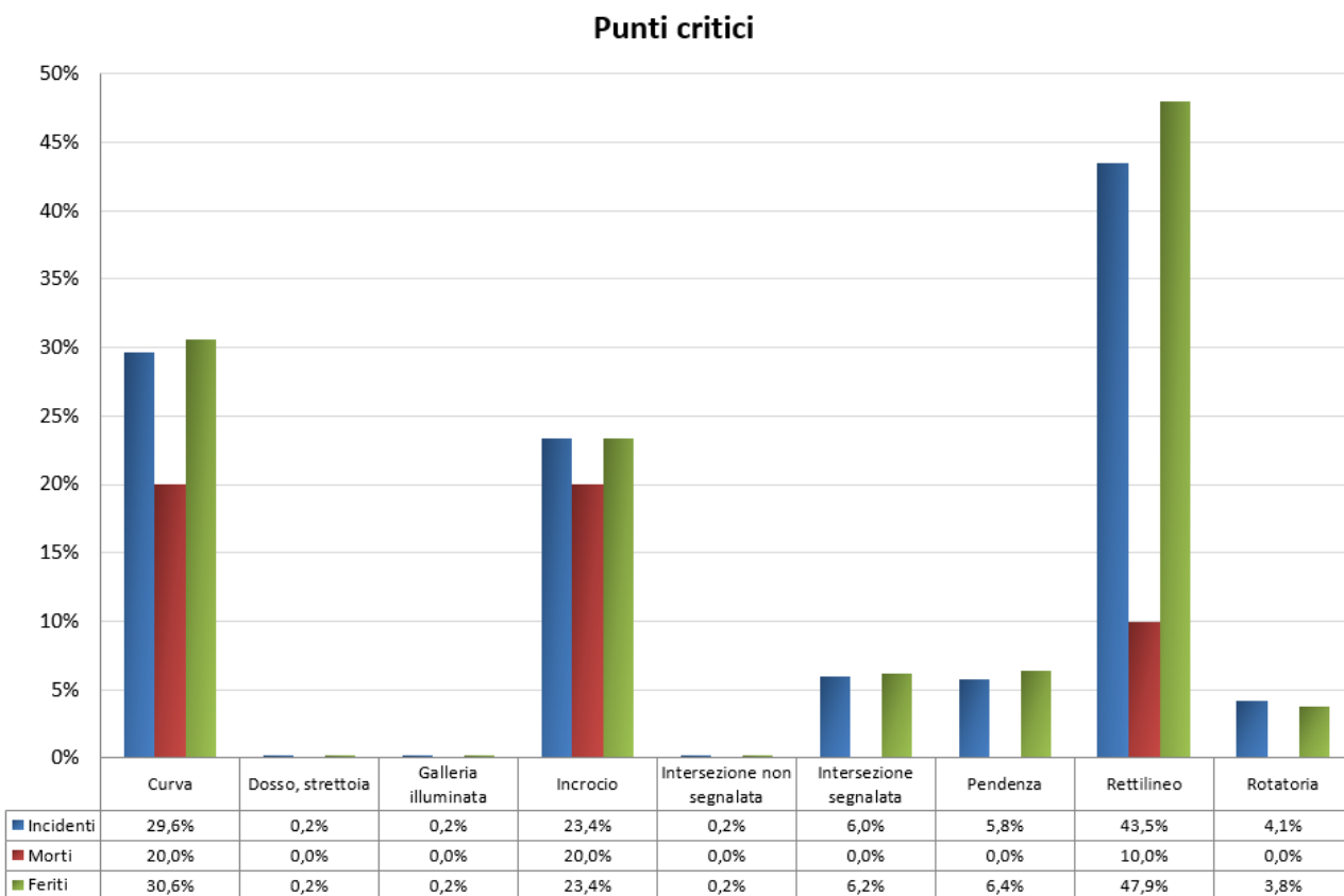
Grafico 27 - Caratteristiche degli incidenti (Quinquennio 2019-2023) – Punti Critici
